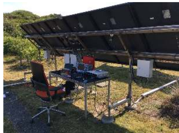
Figuur 2. Buiten-faciliteit voor het testen van vlamboogdetectie bij een echt PV systeem.
